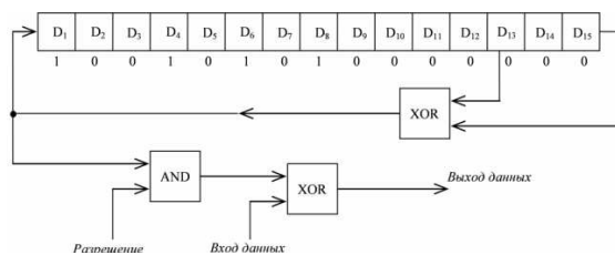
Рис. 1. Генератор последовательности ПСП
