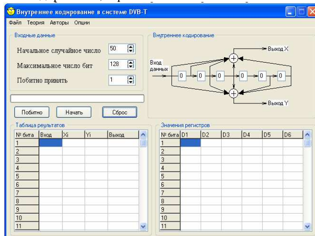
Рис. 6. Окно программы
