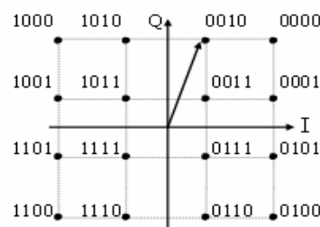
Рис. 4. Сигнальная диаграмма
