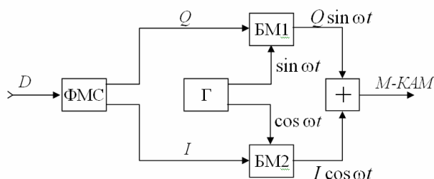
Рис. 3. Схема модуляции
